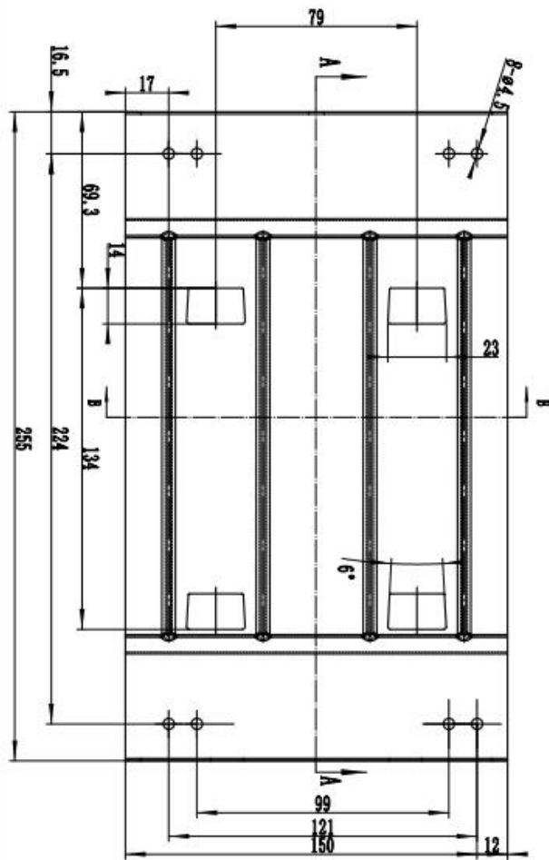
挂板 1 尺寸图
