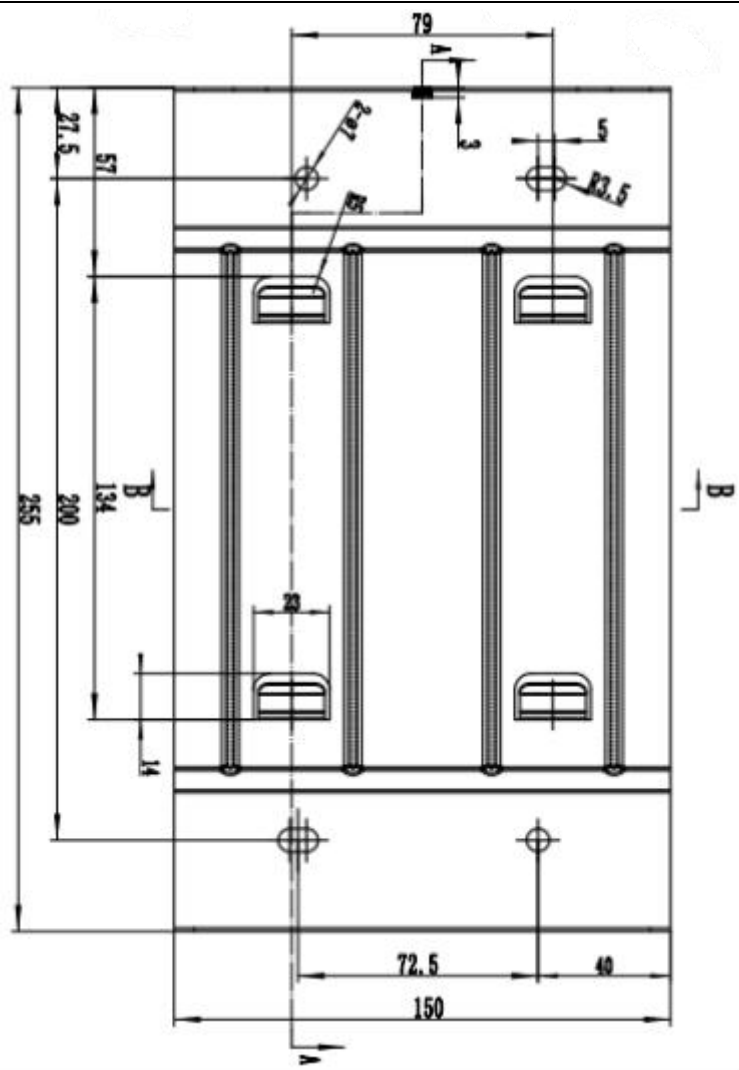
挂板 2 尺寸图
